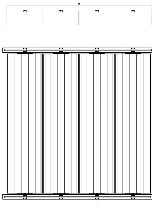
LOUVER 입면도 VERTICAL TYPE
