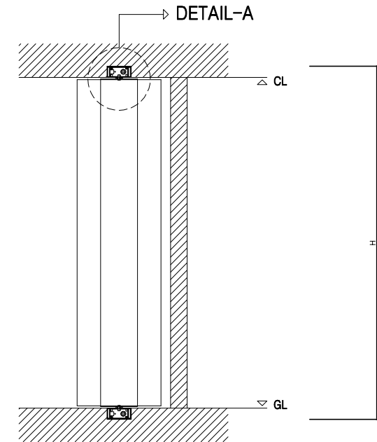
LOUVER 단면도 VERTICAL TYPE
